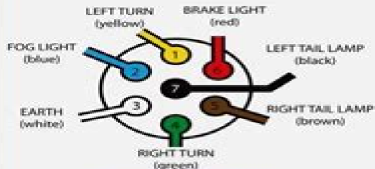
7pin Socket Wiring 12N
