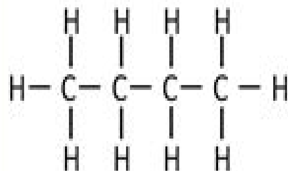
Butane
