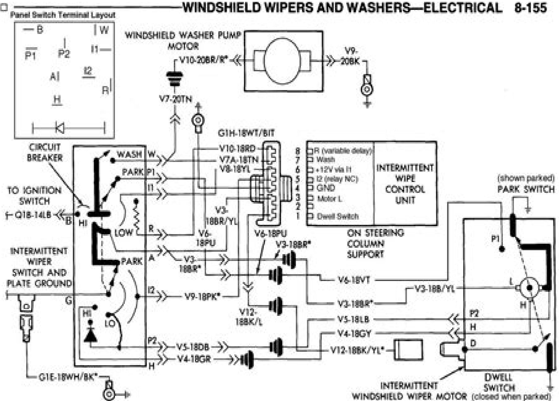
Fig. 25—Intermittent Wipe Wiring Schematic
