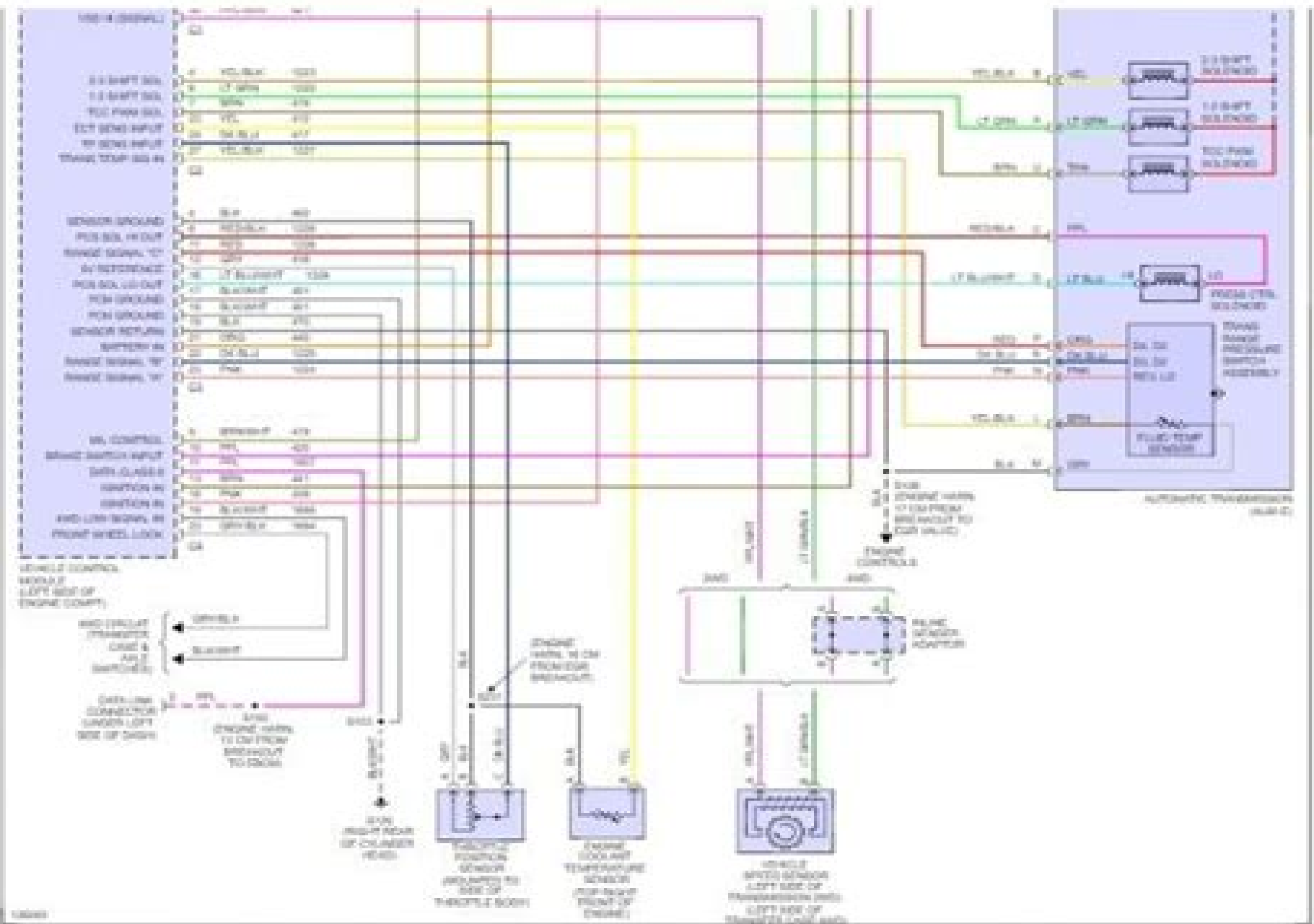
Fig 2: 5.7L VIN R, A/T Circuit, 4L60-E
