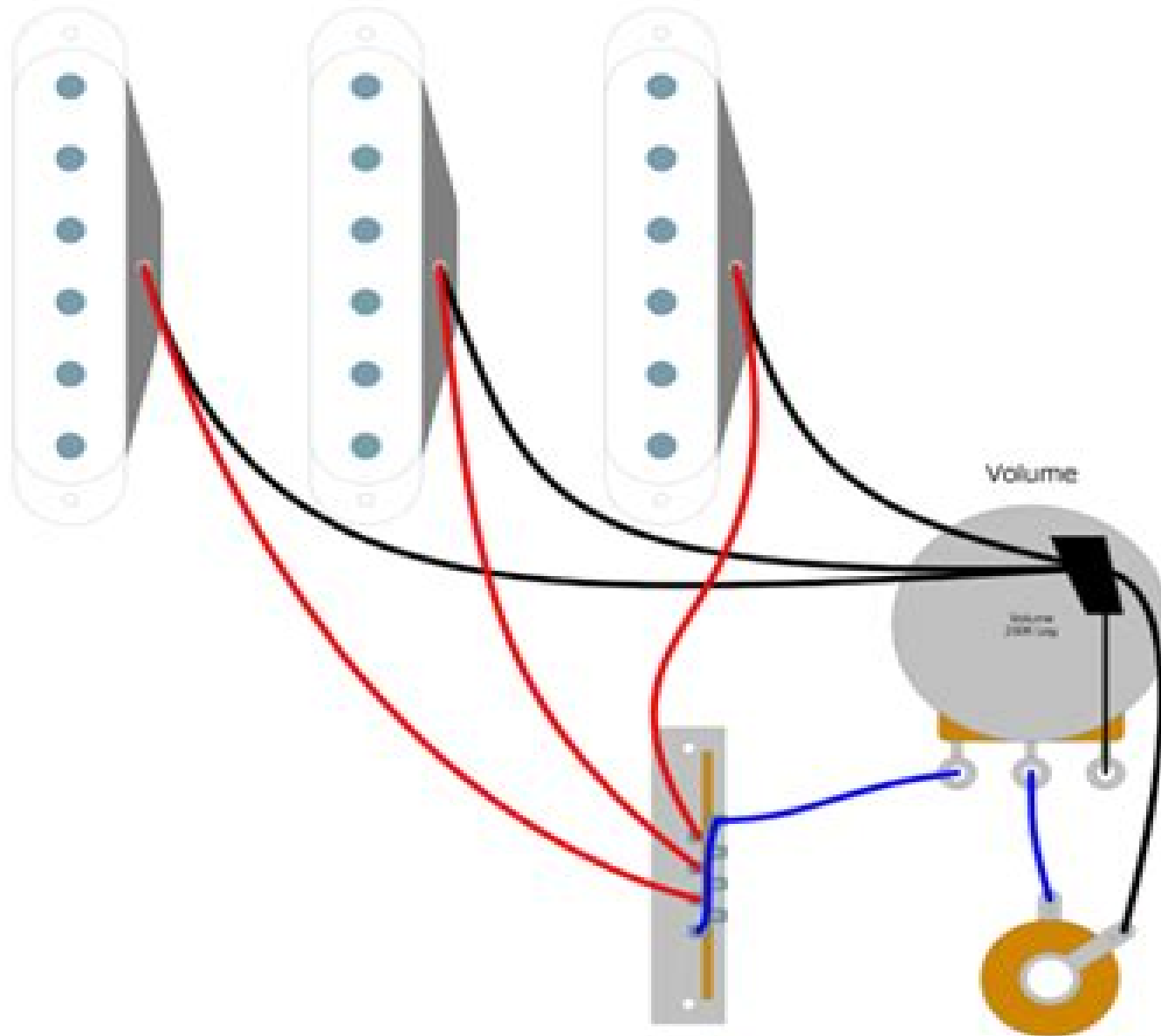
5 Way Switch
