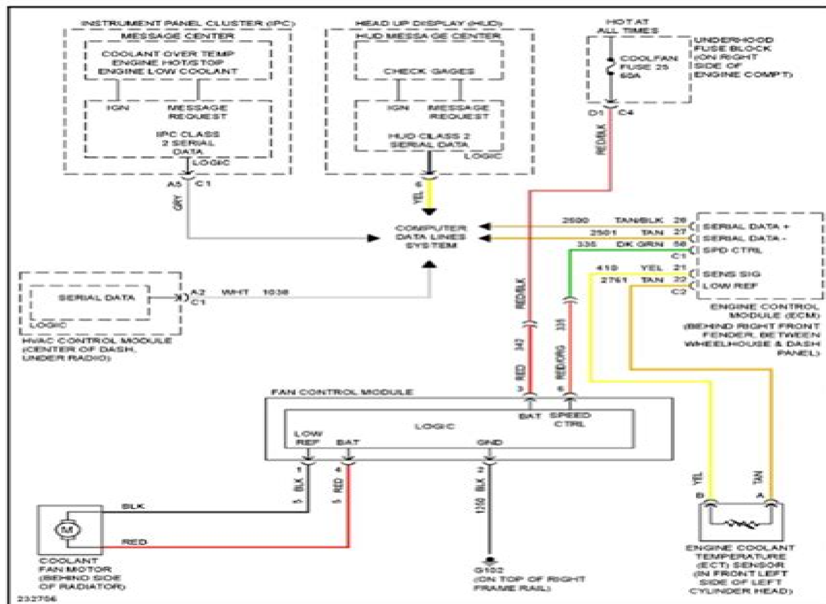
Fig. 15: Cooling Fan Circuit
