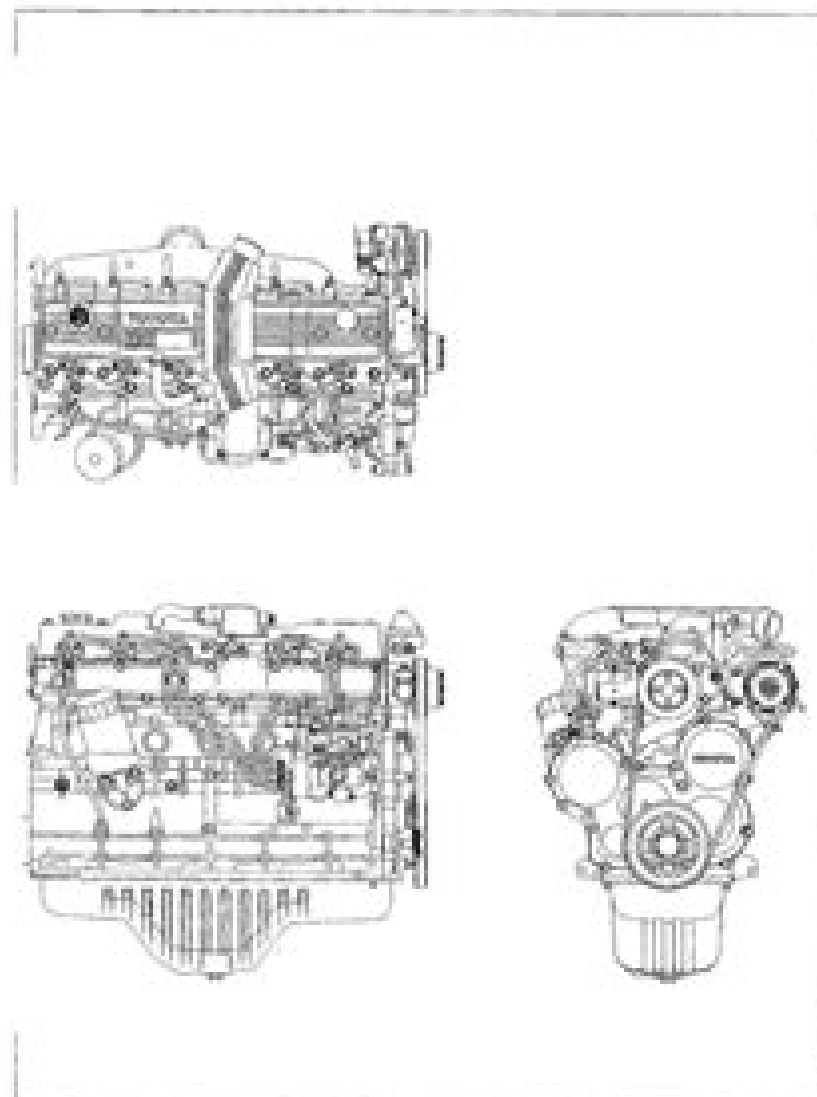
vistas exteriores del motor 132
