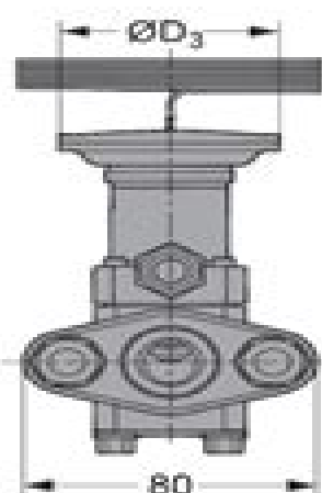
TE12 и 20 - Угловой вентиль под пайку Вес: TE12: 1.5 кг TE20: 1.6 кг
