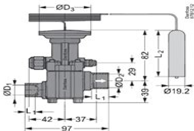
TE12 и 20 - Прямой вентиль под пайку Вес: TE12: 1.5 кг TE20: 1.7 кг
