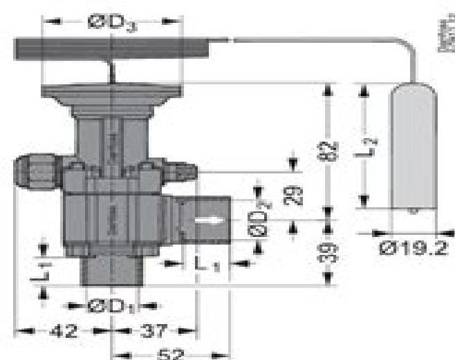
TE12 и 20 - Угловой вентиль под пайку Вес: TE12: 1.5 кг TE20: 1.6 кг
