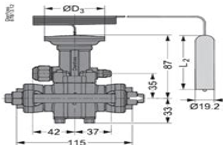
TE12 - Прямой вентиль, фланцы под пайку Вес: Без фильтра: 2.3 кг
